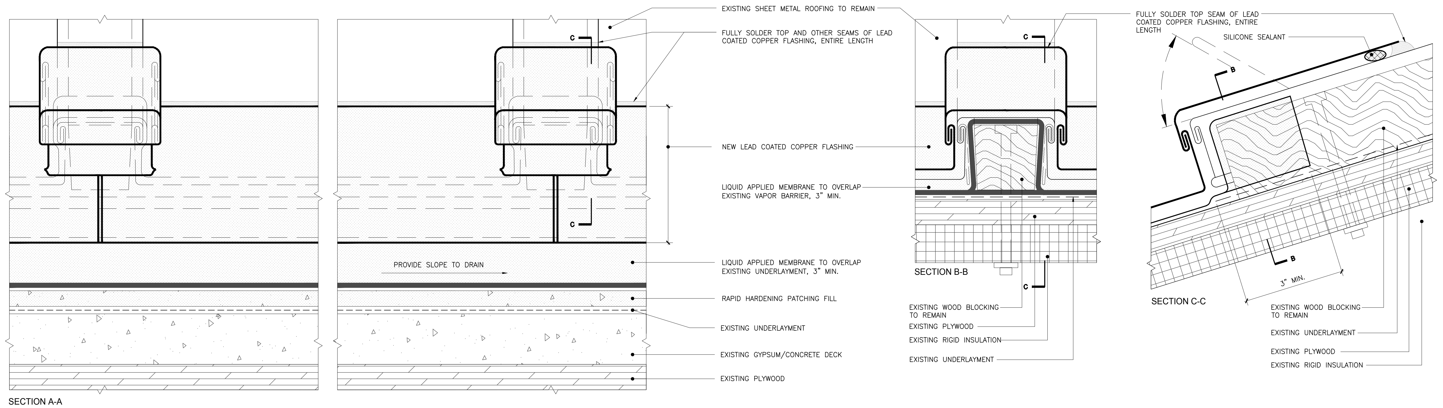
SECTION A-A
